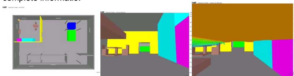
Figuur 6: a. bovenaanzicht van een industrieel gebouw met kantoor en indicatie van brandbronnen; b. situatie voor ontbranding, zicht op het kantoor tegenover de deuropening; c. rooklaag na 600 s, grenslaag met concentratie roetmassa van 24 mg/m 3 , doTINGScoëfficiënt: 0,27 m -1 , zicht: 30 m [10]
